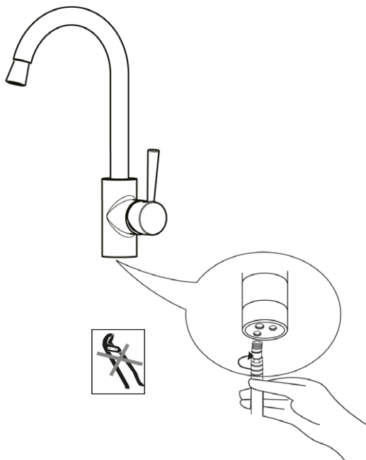
Kuva 1: Liitosletkujen asentaminen.
