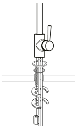
Fig. 2: Montering på benkeplate (tykk).
