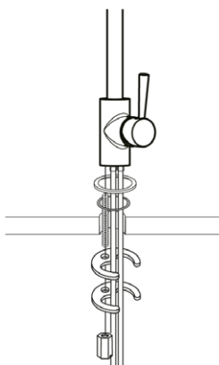
Kuva 2: Asennus työtasoon (paksu).
