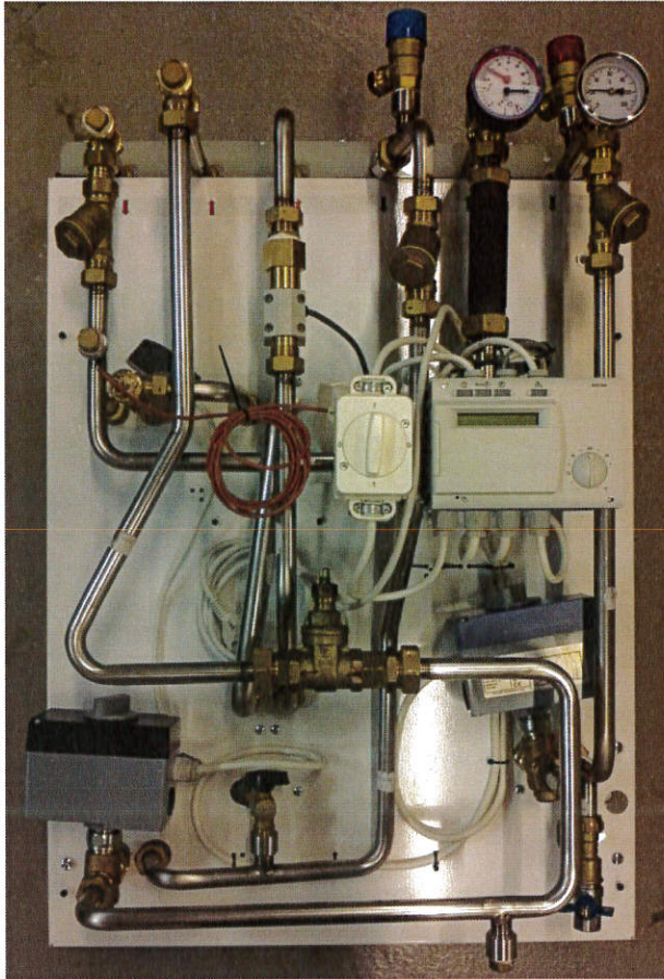
Figur 1. Fjärrvärmecentralen Sirius
