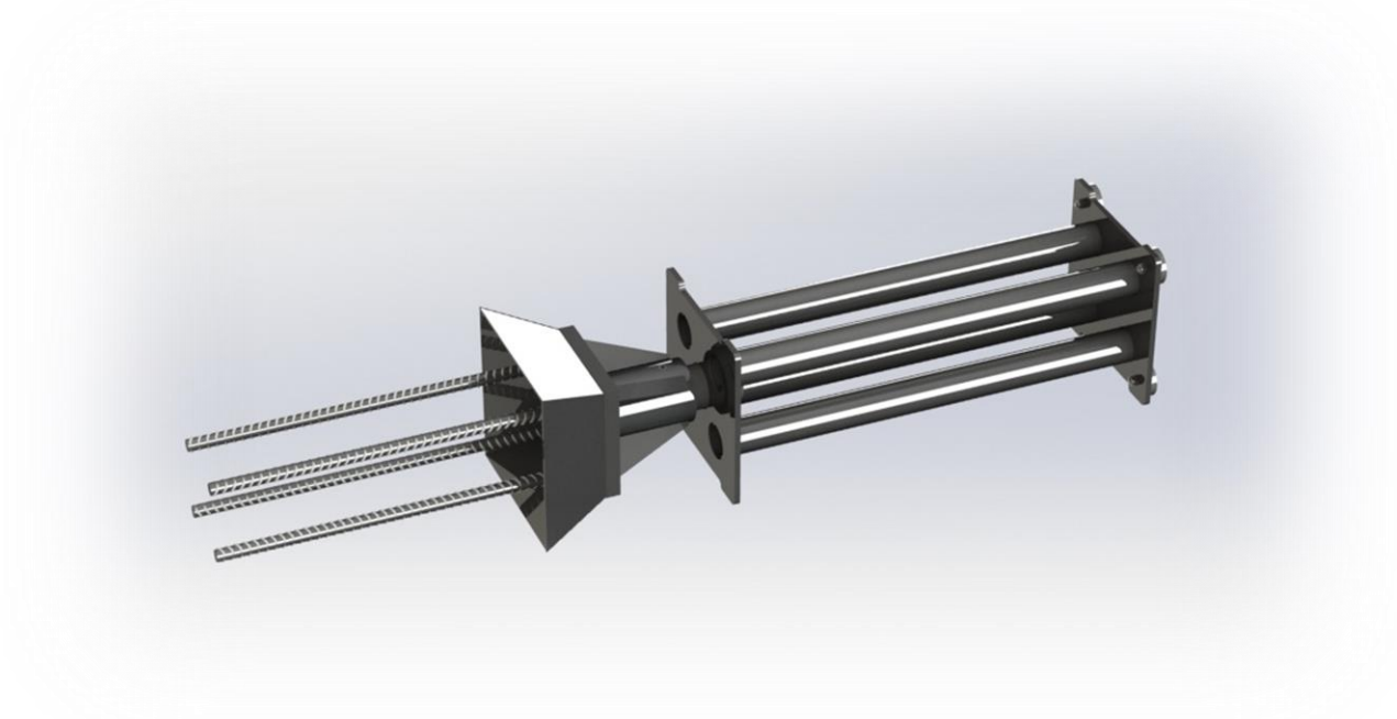
Bild 5. Bergsko med gjutfixtur
