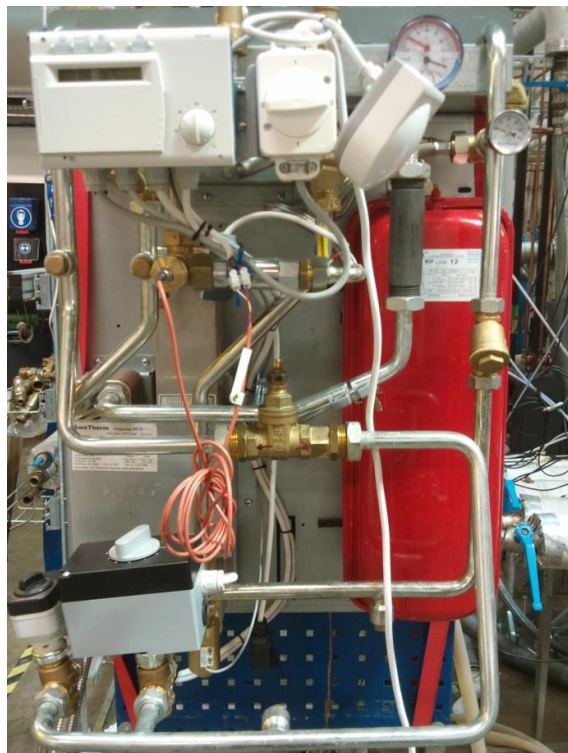
Figur 1. Fjärrvärmecentralen Villaprefab RFS-TPD
